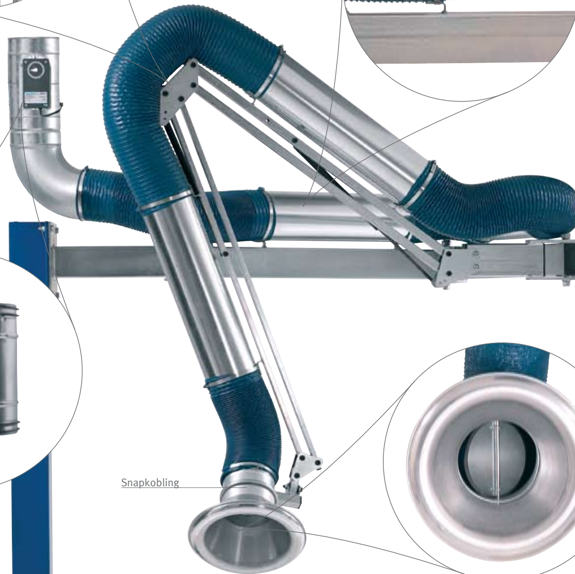
Fleksibelt drejeled med tætsluttende spjæld
